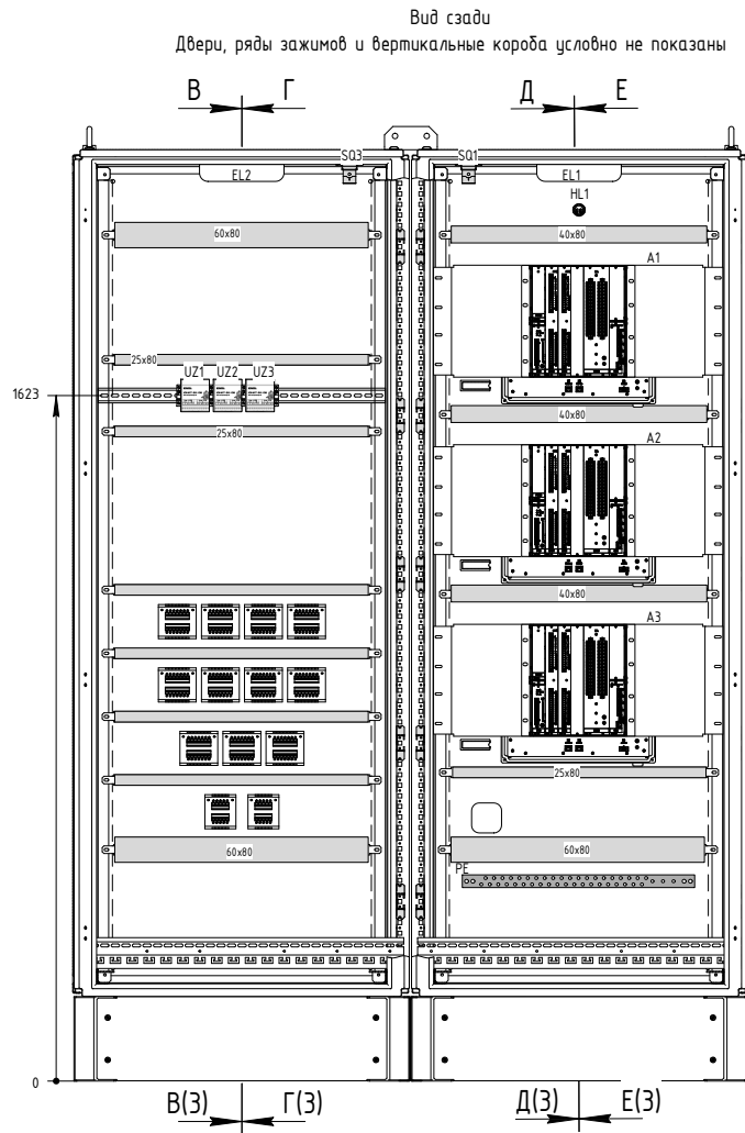
Рисунок В.2 – Чертеж общего вида (часть 2)
